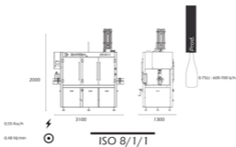
RIEMPITRICE ISOBARICA + TAPPATORE FUNGO + GABBIEATTATRICE Isobaric filler + champagne corker + wire-hooder
